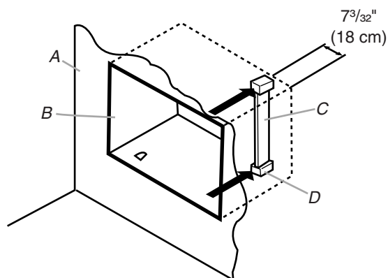
A. Mur B. Avant de la gaine murale C. Plaque de séparation D. Cales de support
