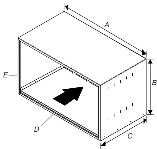
A. Width (W) B. Height (H) C. Depth (D) D. Horizontal insulation strip E. Vertical insulation strip
